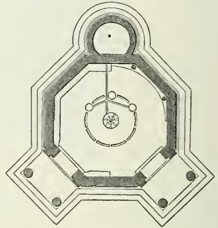
2368 Grundrifs. (Zu Seite 2112.)
