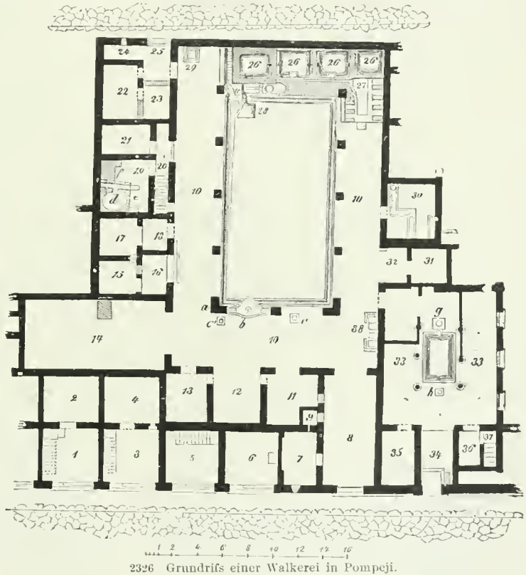
2326 Grundriss einer Walkerei in Pompeji.
