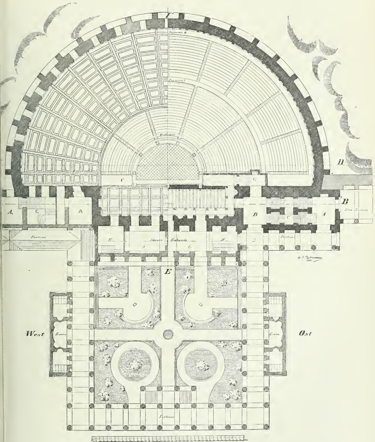
1824 Grundriss vom Odeon des Herodes Atticus zu Athen, Rekonstruktion von Tuckermann. (Zu Seite 1744.)
