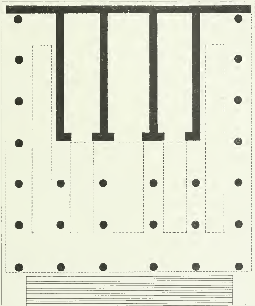
1597 Grundriß des Capitolinischen Jupitertempels. (Zu Seite 1476.)
